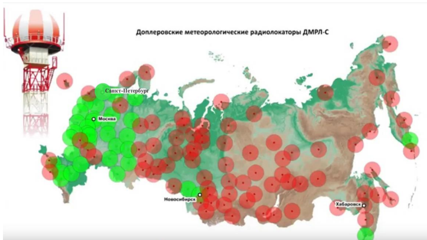
Рисунок 2. Схема расположения ДМРЛ-С на территории РФ (зеленые круги – введенные в эксплуатацию, красные круги неустановленные или нефункционирующие позиции по состоянию на 1 квартал 2018 г.)
