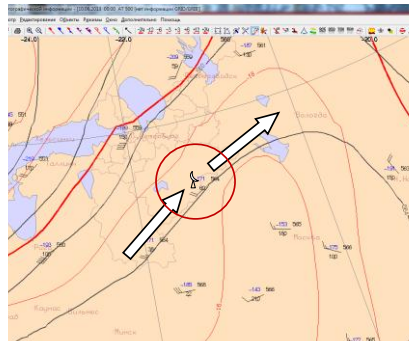
Рисунок 12. Карта абс. топографии изобарической поверхности 500 мб за 00:00 UTC 10.06.2013 в районе Валдая
